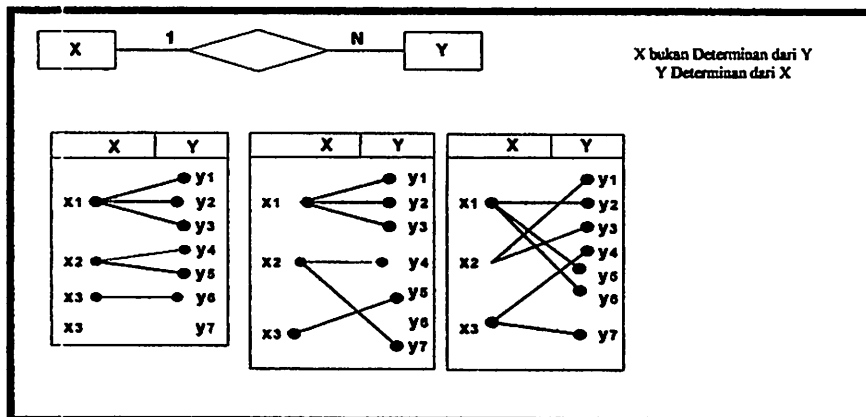
Gambar 2.5. Diagram dan contoh pemunculan hubungan 1:N
