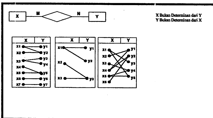
Gambar 2.7. Diagram dan contoh pemunculan hubungan M:N
