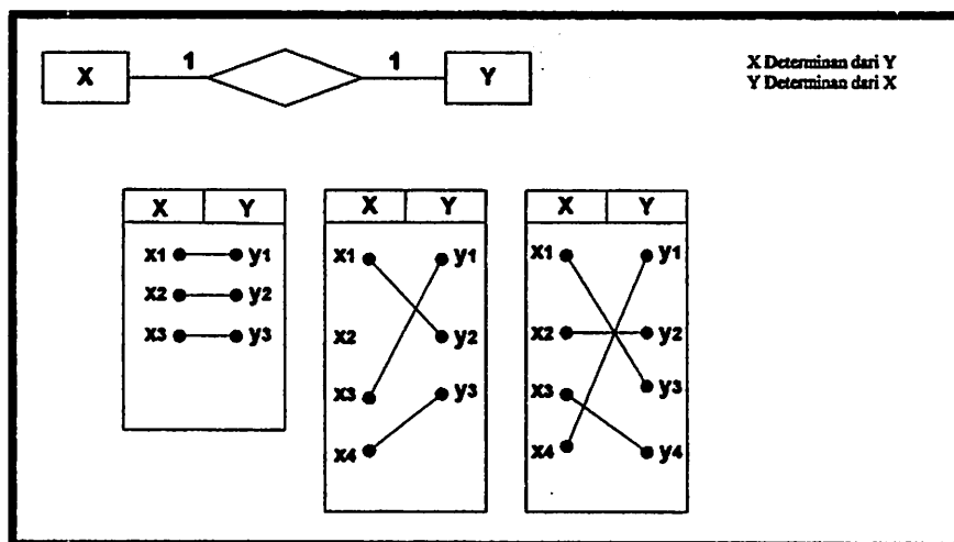
Gambar 2.4. Diagram dan contoh pemunculan hubungan 1:1
