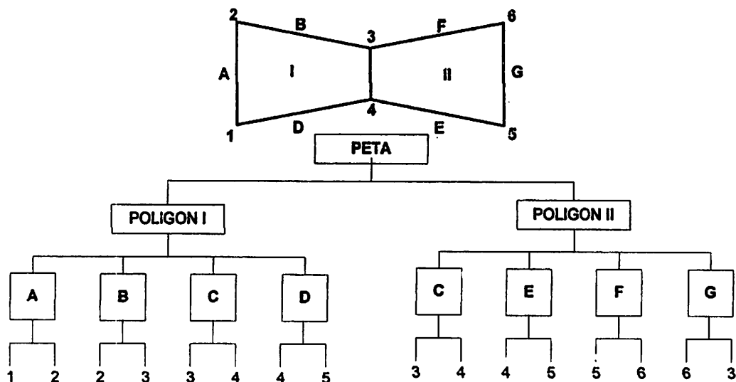
Gambar 2.2. Struktur database Hirarki
