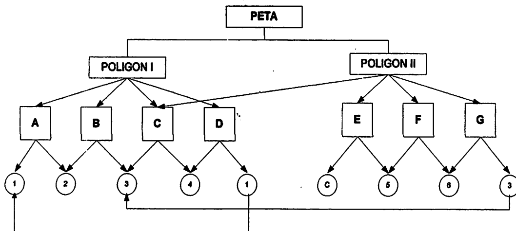
Gambar 2.3. Struktur Database Network
