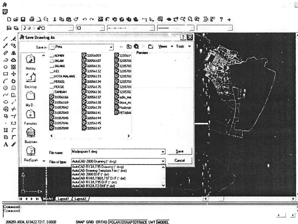
Gambar 2.15. Eksport Data
