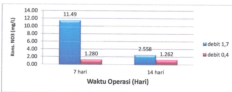
Gambar 4.14 Hubungan Konsentrasi Akhir NO 3 (mg/l) Terhadap Waktu Operasi ( Reaktor Filter Aerobik)
