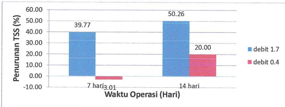
Gambar 4.12 Grafik Persentase Penurunan Nilai Konsentrasi TSS Terhadap Waktu Operasi ( Reaktor Filter Aerobik)
