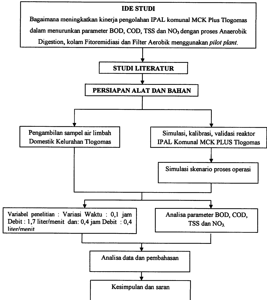
Gambar 3.2. Kerangka Penelitian
