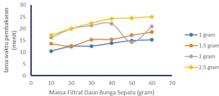
Gambar 5. Hubungan Antara Massa Filtrat Daun Bunga Sepatu dan Massa Carbopol -940 terhadap Lama Waktu Pembakaran
