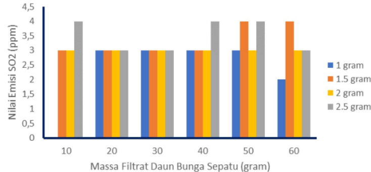
Gambar 4. Hubungan Antara Massa Filtrat Daun Bunga Sepatu dan Massa Carbopol-940 terhadap Nilai SO 2
