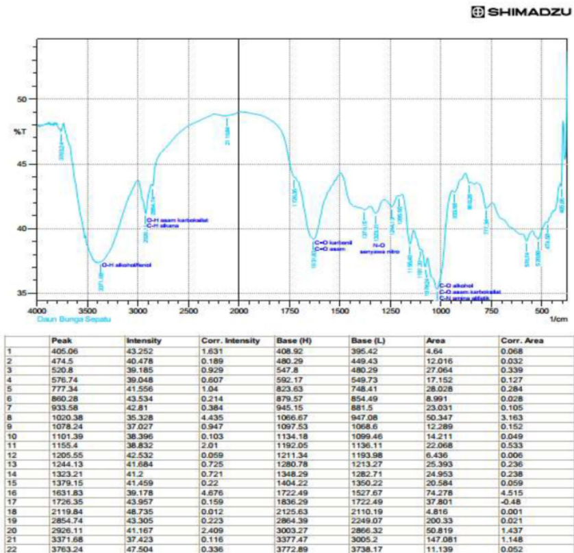
Gambar 2 Analisis gugus fungsi Daun bunga sepatu menggunakan FTIR
