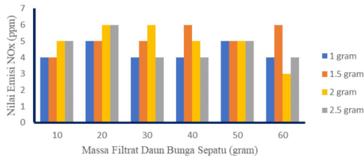
Gambar 3. Hubungan Antara Massa Filtrat Daun Bunga Sepatu dan Massa Carbopol-940 terhadap Nilai NOx
