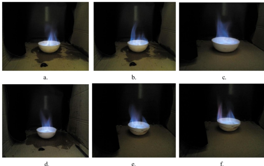
Gambar 8. Nyala api Sterno Gel Daun Bunga Sepatu dengan Massa Filtrat Daun Bunga Sepatu a)10 gram, b) 20 gram, c) 30 gram, d) 40 gram, e) 50 gram, dan f) 60 gram.
