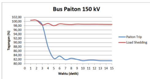
Gambar 10. Grafik Perubahan Tegangan 150 kV
