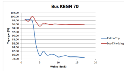
Gambar 11. Grafik Perubahan Tegangan Bus 70 kV
