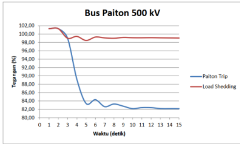
Gambar 9. Grafik Perubahan Tegangan Bus 500 kV
