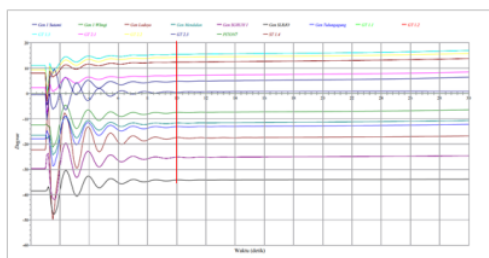
Gambar 14. Grafik Perubahan Sudut Rotor Setelah Load Shedding
