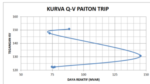
Gambar 17. Kurva Q-V Bus Paiton 150 Paiton Trip
