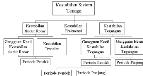
Gambar 1. Kestabilan Sistem Tenaga Listrik [1]
