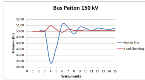
Gambar 12. Grafik Perubahan Frekuensi
