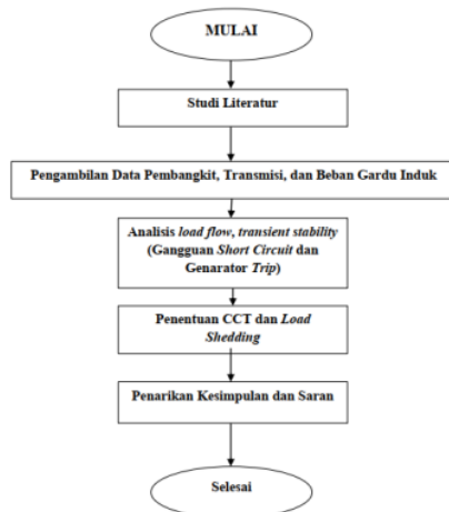
Gambar 3. Diagram Alir Metode Penelitian
