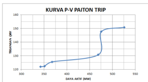
Gambar 15. Kurva P-V Bus Paiton 150 kV Paiton Trip
