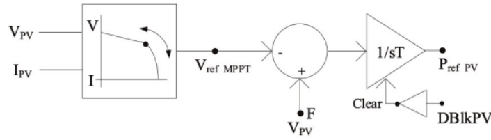
Fig. 5. MPPT controller.
