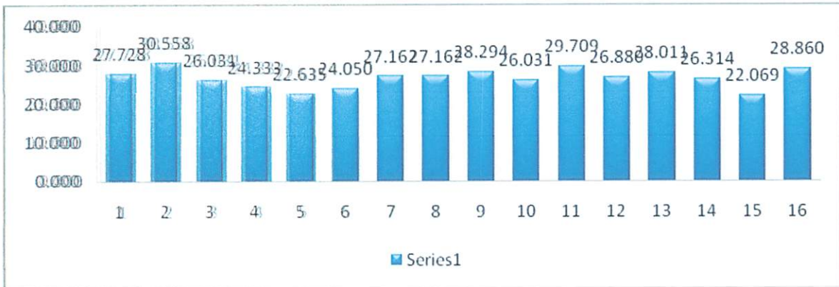
Grafik 5.3 untuk Kuat tekan Beton (Variasi 30%)
