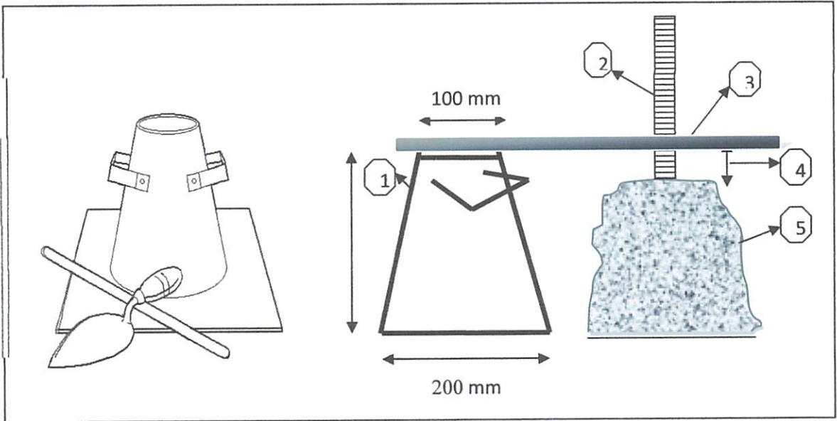
Gambar 3.1 Peralatan uji slump dan pengujian nilai slump
