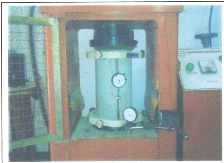
Gambar 5.4. Pengujian Modulus Elastisitas
