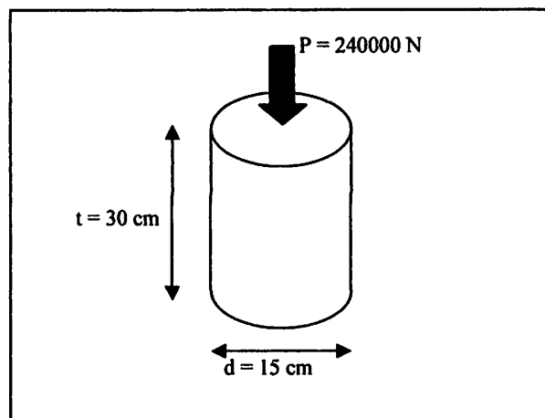
Gambar 5.1 Pengujian Kuat Tekan
