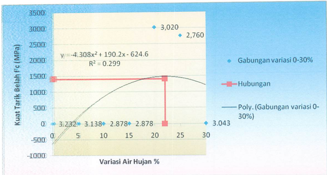
Grafik 5.6 Analisa Regresi Untuk Kuat Tarik Belah (Variasi 0 – 30%)
