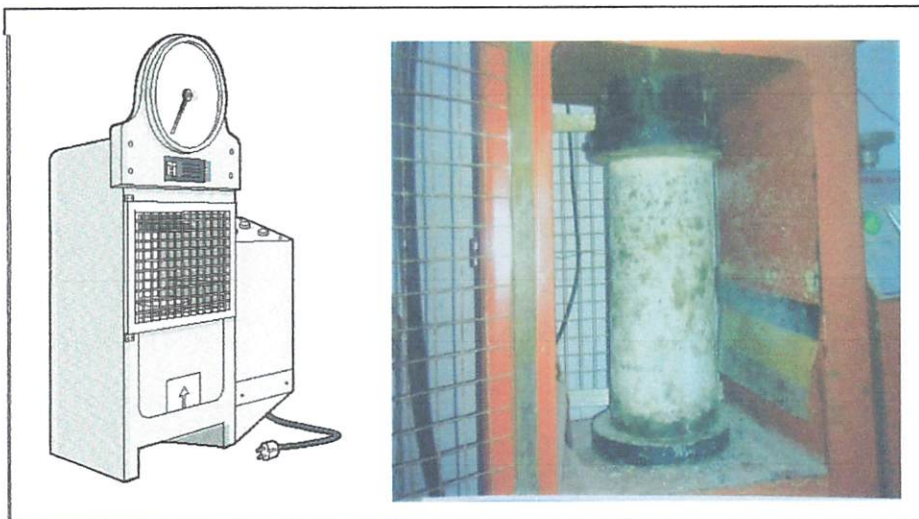
Gambar 3.3 Mesin uji Kuat tekan dan pengujian Kuat Tekan
