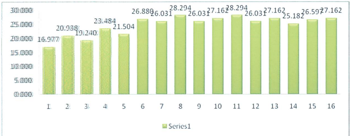
Grafik 5.2 untuk Kuat tekan Beton (Variasi 20%)
