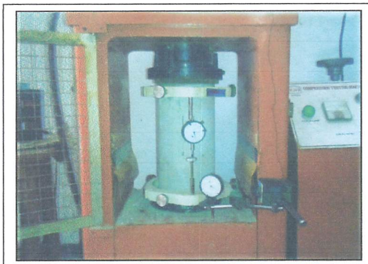
Gambar 3.7 Pengujian Modulus Elastisitas
