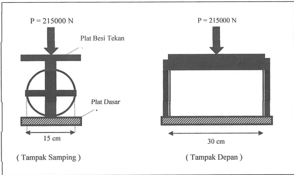
Gambar 5.2 Pengujian Kuat Tarik Belah Beton
