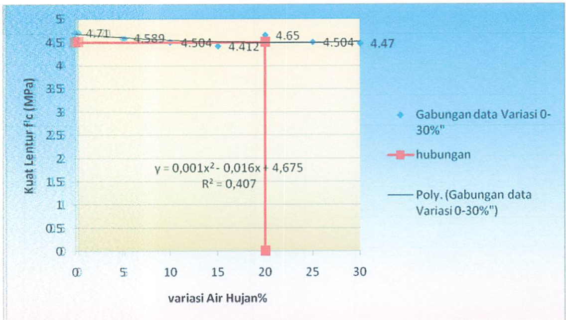
Grafik 5.7 Analisa Regresi Untuk Kuat Tarik Lentur (Variasi 0 – 30%)
