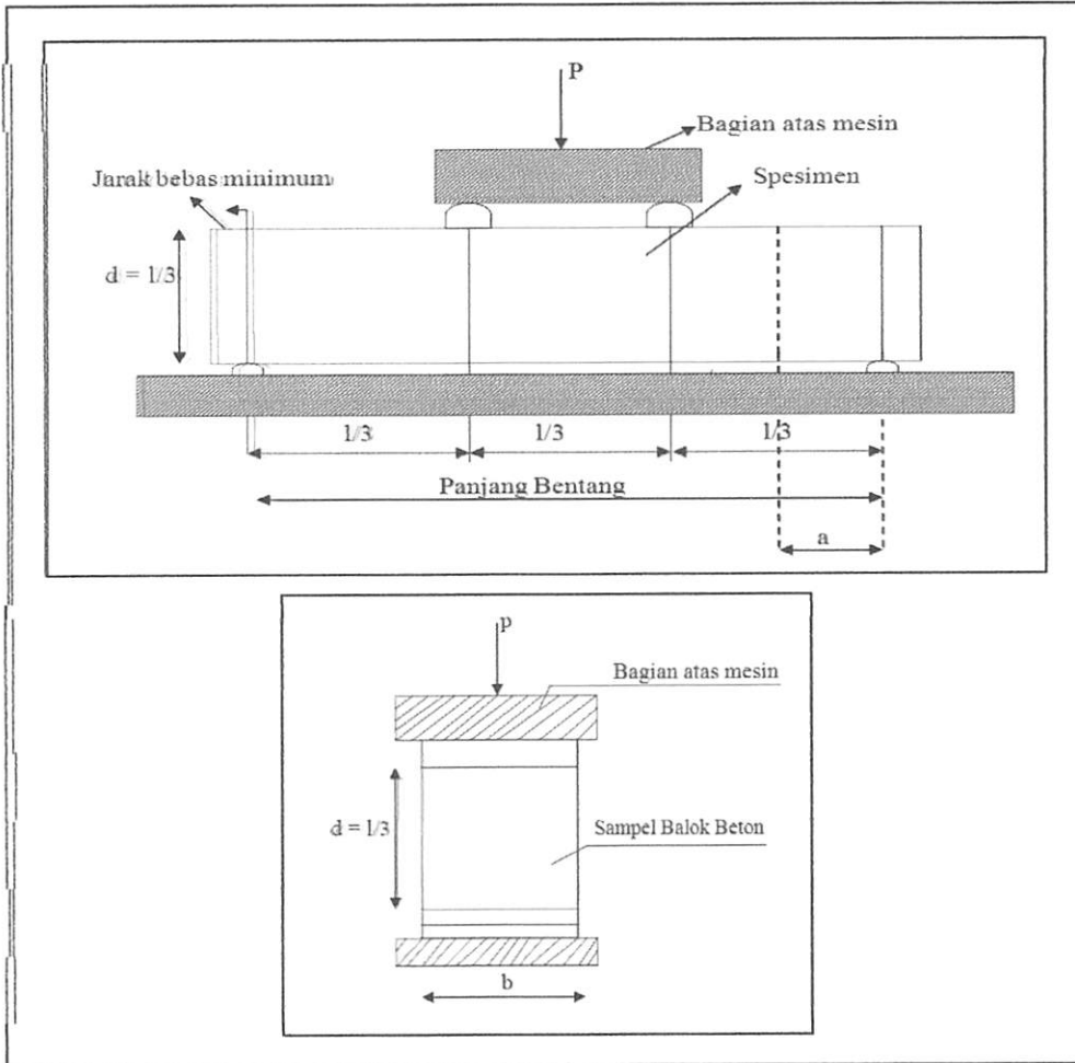
Gambar 3.5. Ilustrasi Kuat Lentur Balok dilihat dari samping (atas)
