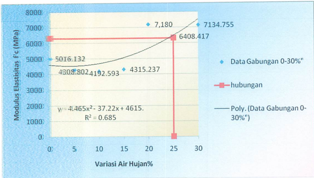
Grafik 5.8 Analisa Regresi Untuk Modulus Elastisitas (Variasi 0 – 30%)
