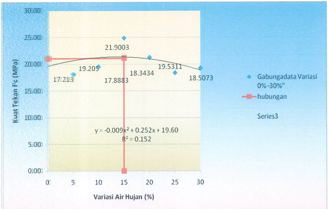
Grafik 5.5 Analisa Regresi Untuk Kuat Tekan (Variasi 0 – 30%)
