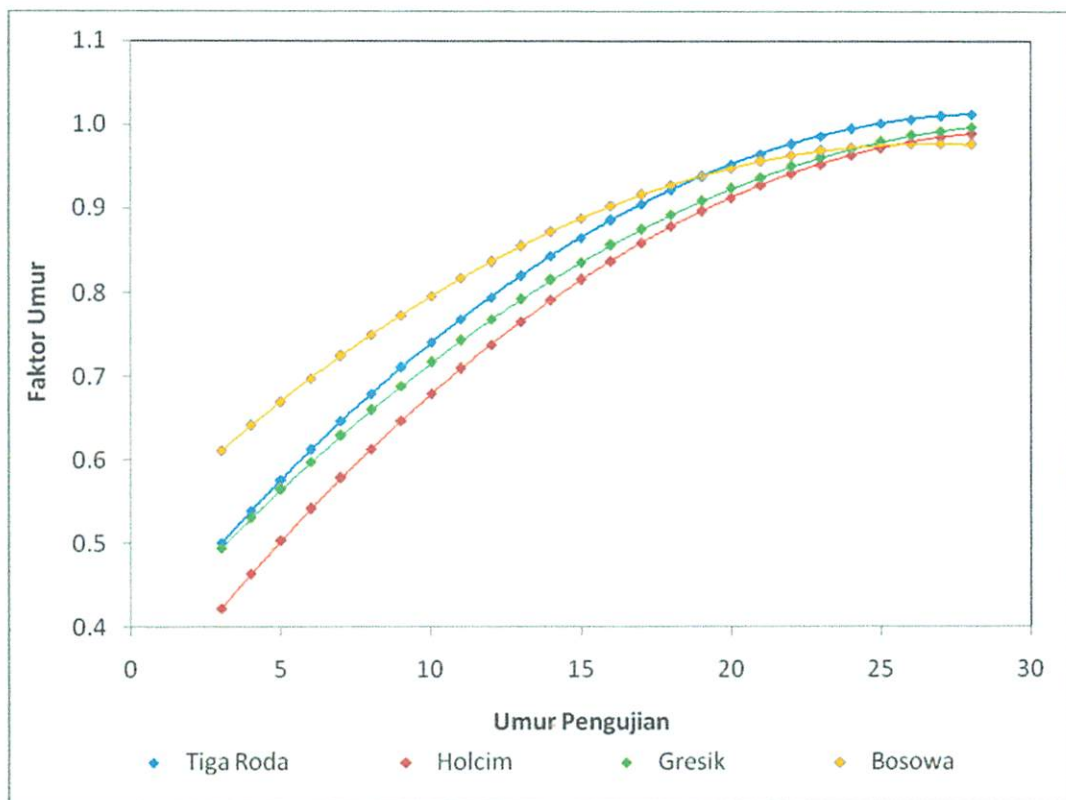
Gambar 5.4. Grafik Hubungan antara Umur Pengujian dengan Faktor Umur beton f'c 35 MPa menggunakan semen Tiga Roda dengan Semen Semen Holcim PCC, semen Gresik jenis PPC, dan semen Bosowa jenis PCC
