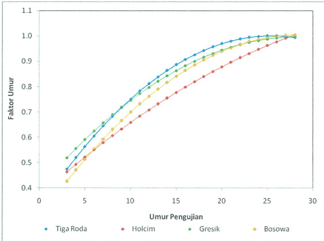
Gambar 5.3. Grafik Hubungan antara Umur Pengujian dengan Faktor Umur beton f'c 20 MPa menggunakan semen Tiga Roda dengan Semen Holcim jenis PCC, semen Gresik jenis PPC dan semen Bosowa jenis PCC
