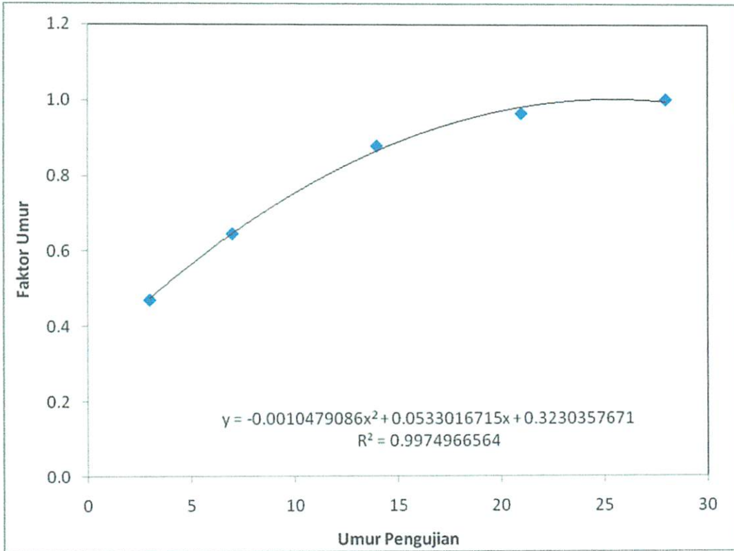
Gambar 5.1. Grafik Hubungan antara Umur Pengujian dengan Faktor Umur beton f'c 20 MPa menggunakan semen Tiga Roda jenis PCC
