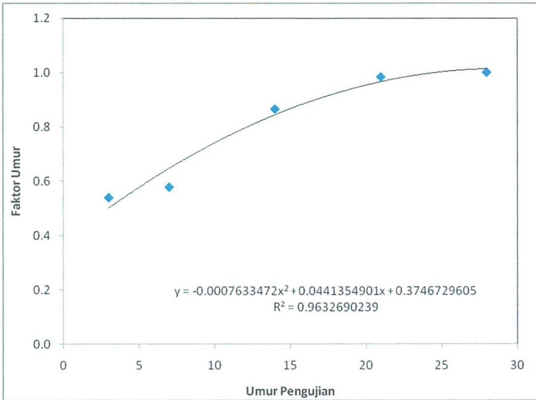
Gambar 5.2. Grafik Hubungan antara Umur Pengujian dengan Faktor Umur beton f'c 35 MPa menggunakan semen Tiga Roda PCC
