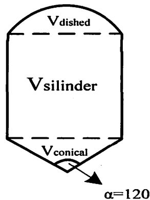
Gambar 6.1. Volume total dari Reaktor Esterifikasi
