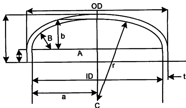
Gambar 6.2. Dimensi tutup atas standart dished reaktor
