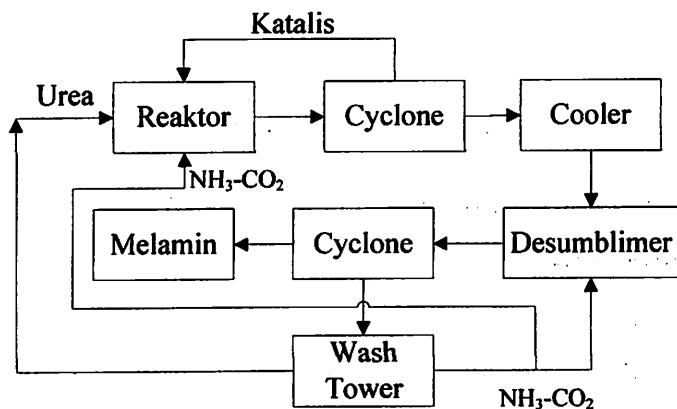
Gambar 2.1.3.3. Blok Diagram Proses Pembuatan Melamin Dengan Proses BASF
