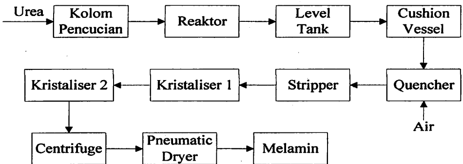
Gambar 2.1.3.2. Blok Diagram Proses Pembuatan Melamin Dengan Proses Nissan
