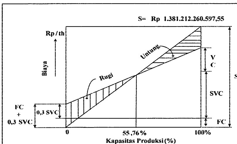
Gambar 11.1. Break Even Point (BEP) Pra Rencana Pabrik Melamin
