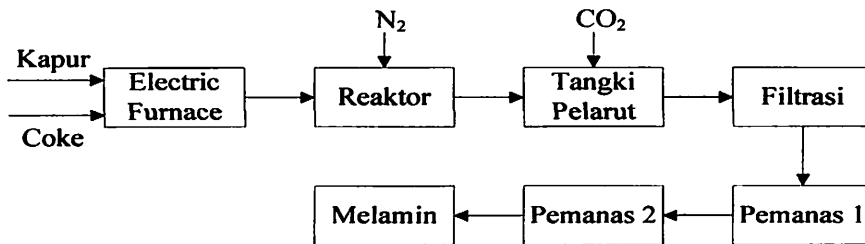
Gambar 2.1.1. Blok Diagram Proses Pembuatan Melamin Dengan Dicyanamida
