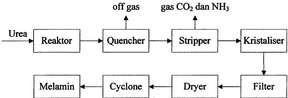
Gambar 2.1.3.1. Blok Diagram Pembuatan Melamin Dengan Proses Montedison
