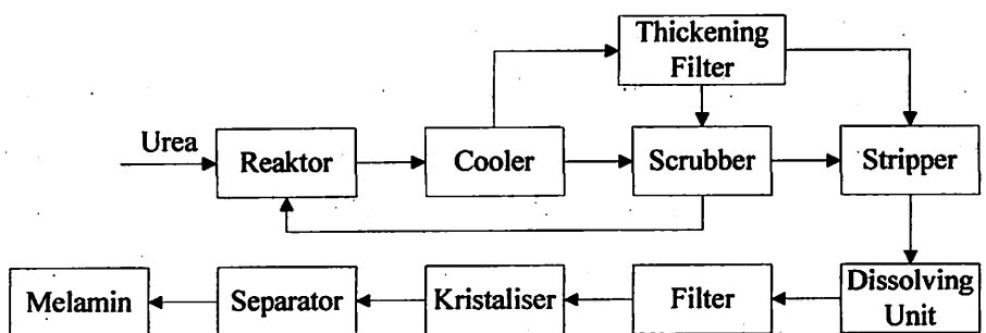
Gambar 2.1.3.4. Blok Diagram Proses Pembuatan Melamin Dengan Proses Stamicarbon
