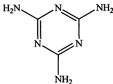
Gambar 1.2. Gugus molekul melamin
