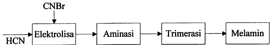
Gambar 2.1.2. Blok Diagram Proses Pembuatan Melamin Dengan HCN
