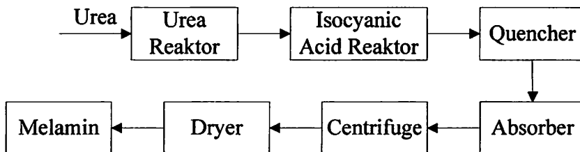
Gambar 2.1.3.5. Blok Diagram Proses Pembuatan Melamin Dengan Proses OSW
