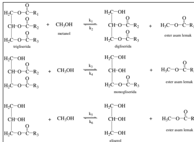
Gambar 2. Tahapan Reaksi Transesterifikasi Trigliserida dengan Metanol
