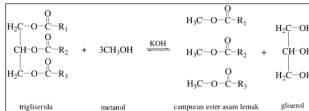
Gambar 1. Reaksi Transesterifikasi Trigliserida dengan Metanol
