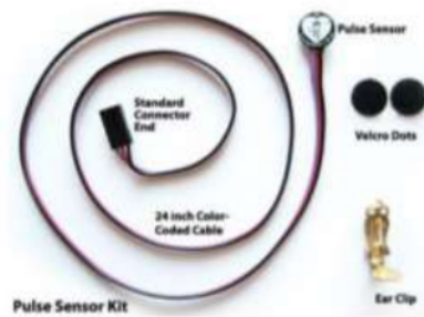
1 Gambar 2.19 Komponen Perangkat Pulse Sensor ( http://pulsesensor.com/ )
