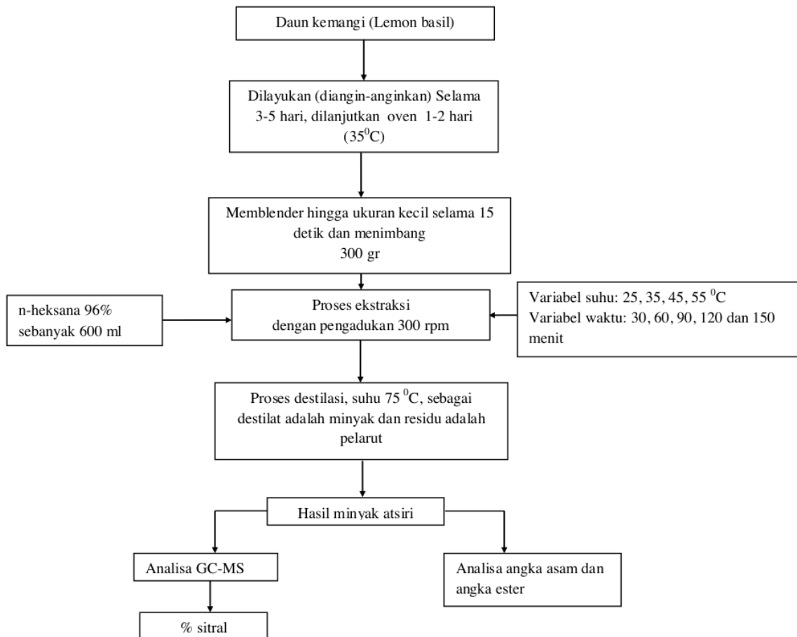
Gambar 1. Kerangka Penelitian Ekstraksi Minyak Atsiri Daun Kemangi
