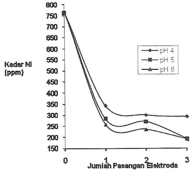
Gambar 7. Hubungan antara kadar nikel (ppm) terhadap pH dan jumlah pasangan elektroda pada suhu proses 55°C dan waktu proses 60 menit
