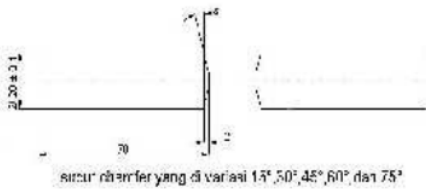
Gambar 1. Dimensi Benda Kerja
