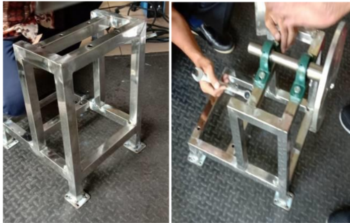
Gambar 4. Pengelasan dan perakitan komponen mesin Perajang
