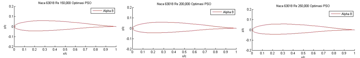
Gambar 8 Geometri Naca 63(3)018 Optimasi PSO Sudut Serang 8^\circ
