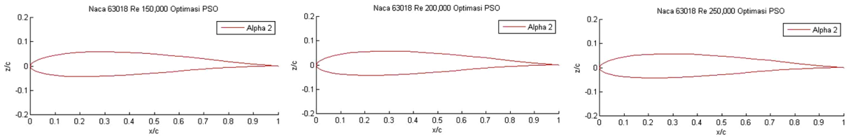
Gambar 5 Geometri Naca 63(3)018 Optimasi PSO Sudut Serang 2^\circ
