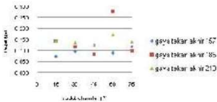
15 Gambar 4. Grafik hubungan antara sudut chamfer, gaya tekan akhir dan kekuatan tarik
