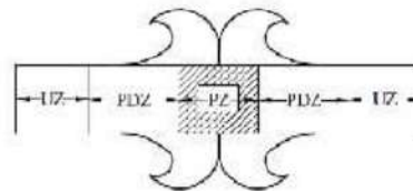
Gambar 6. Penampang melintang dari pengelasan gesek yang menunjukkan daerah UZ ( undeformed zone ), PDZ ( partly deformed zone ) dan PZ ( plasticized zone ) [5]
