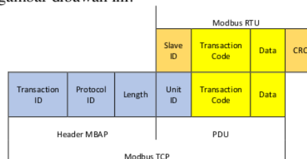
Gambar 6. Format Frame Modbus TCP
