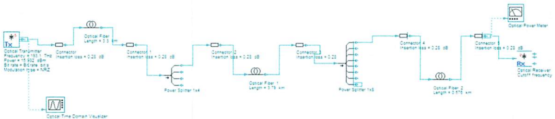
Gambar 4.4 Simulasi Jaringan FTTH di Warungdowo
