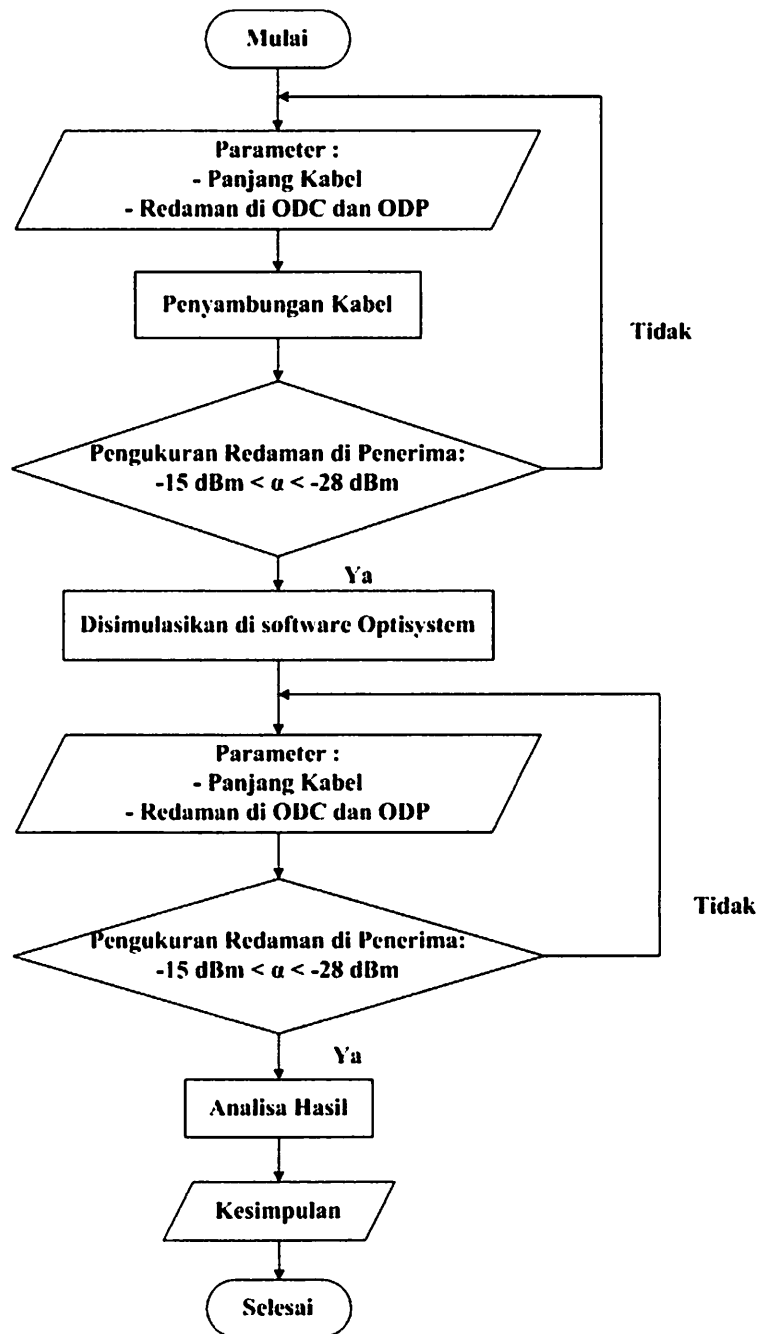
Gambar 3.1 Diagram Alir Perancangan Sistem
