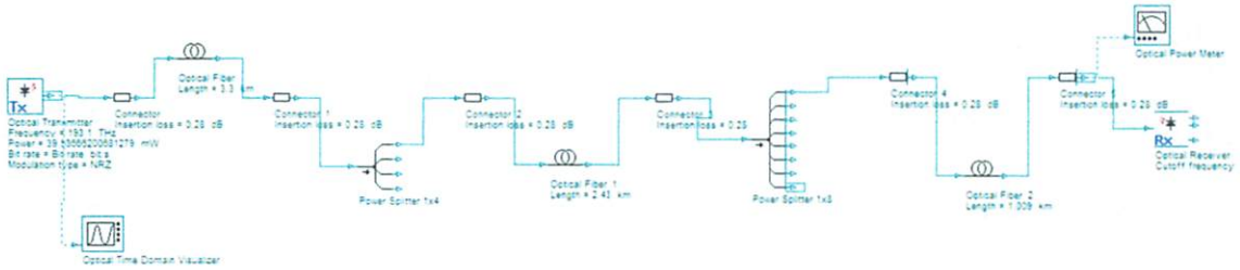
Gambar 4.3 Simulasi Jaringan FTTH di Sidogiri
