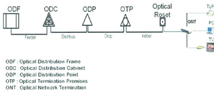
Gambar 3.4 Topologi Jaringan FTTH
