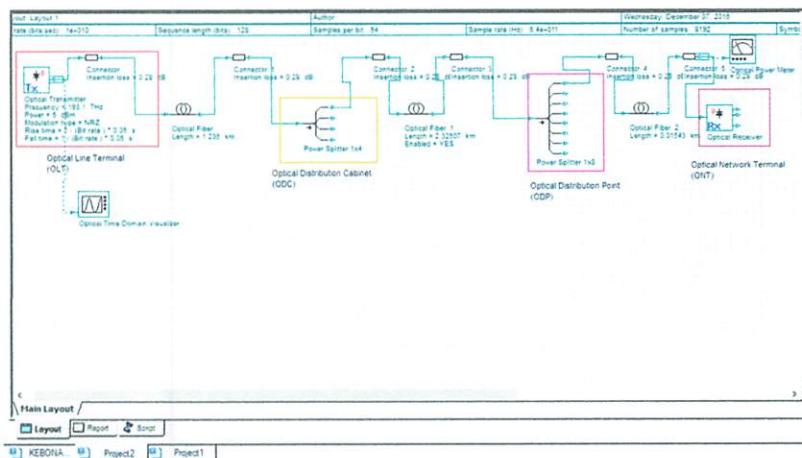
Gambar 3.15 Simulasi siap
