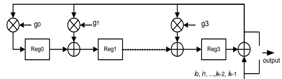
Gambar 2. Rangkaian RS (31, 27) enkoder.
