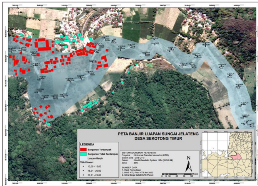
Gambar 12. Peta bangunan terdampak banjir Sungai Jelateng, Desa Sekotong Timur, Kec Lembar.
