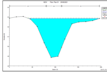
Gambar 5. Tampilan Cross sungai jelatang hasil pemodelan hidraulika
