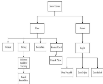
Gambar 2 Struktur Menu
