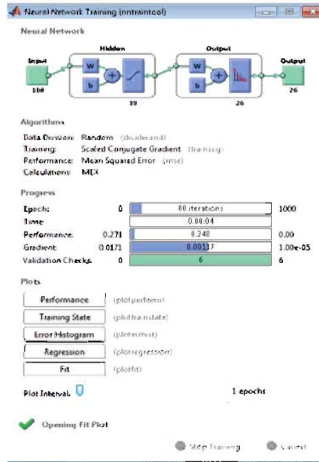
Gambar 2. Tampilan Hasil Pelatihan JST.
