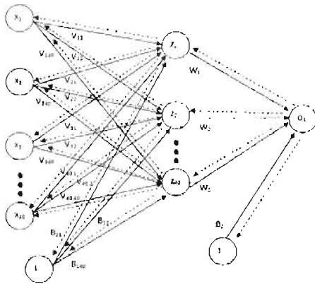
Gambar 1. Arsitektur Backpropagation
