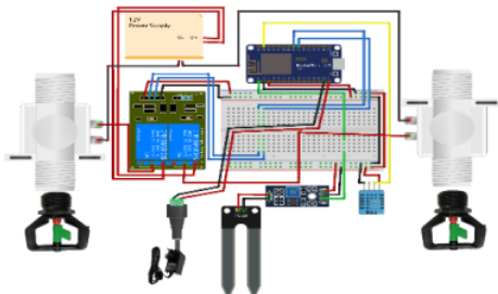
Gambar 11 Desain Alat
