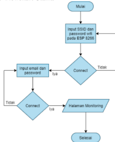
Gambar 8. Flowchart Utama
