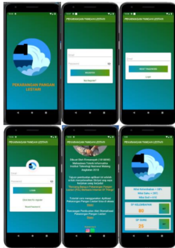
Gambar 14. Tampilan Aplikasi
