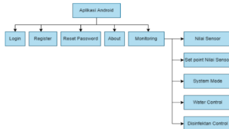
Gambar 7. Struktur Menu
