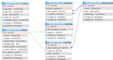
Gambar 1. Perancangan Database
