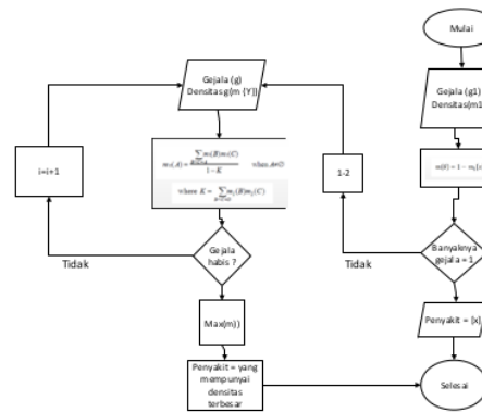
Gambar 4. Mesin Inferensi Dempster shafer
