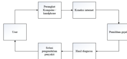
Gambar 1 Desain sistem
