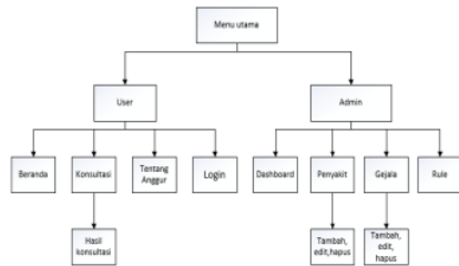
Gambar 2 Struktur menu
