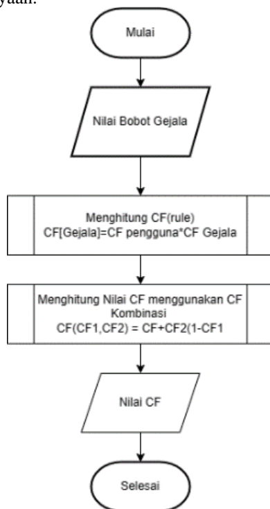
Gambar 3 Flowchart dari Metode Certainty Factor
