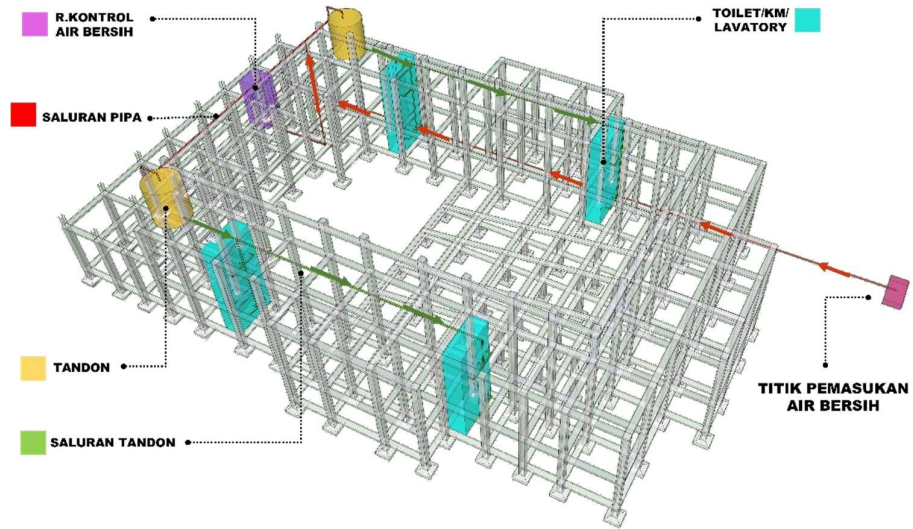
Gambar 5.5. Konsep Utilitas
