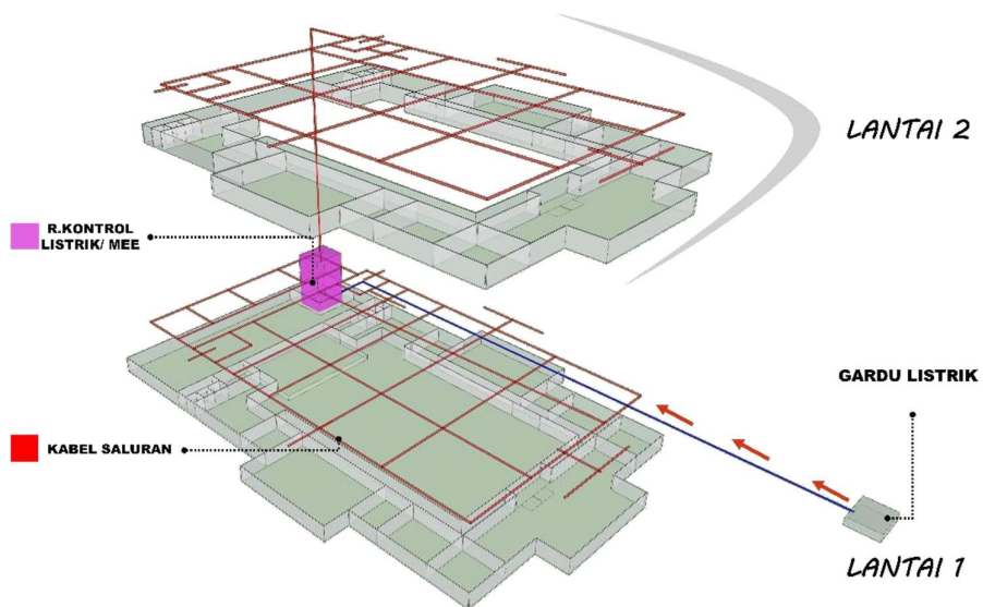
Gambar 5.6. Konsep Utilitas
