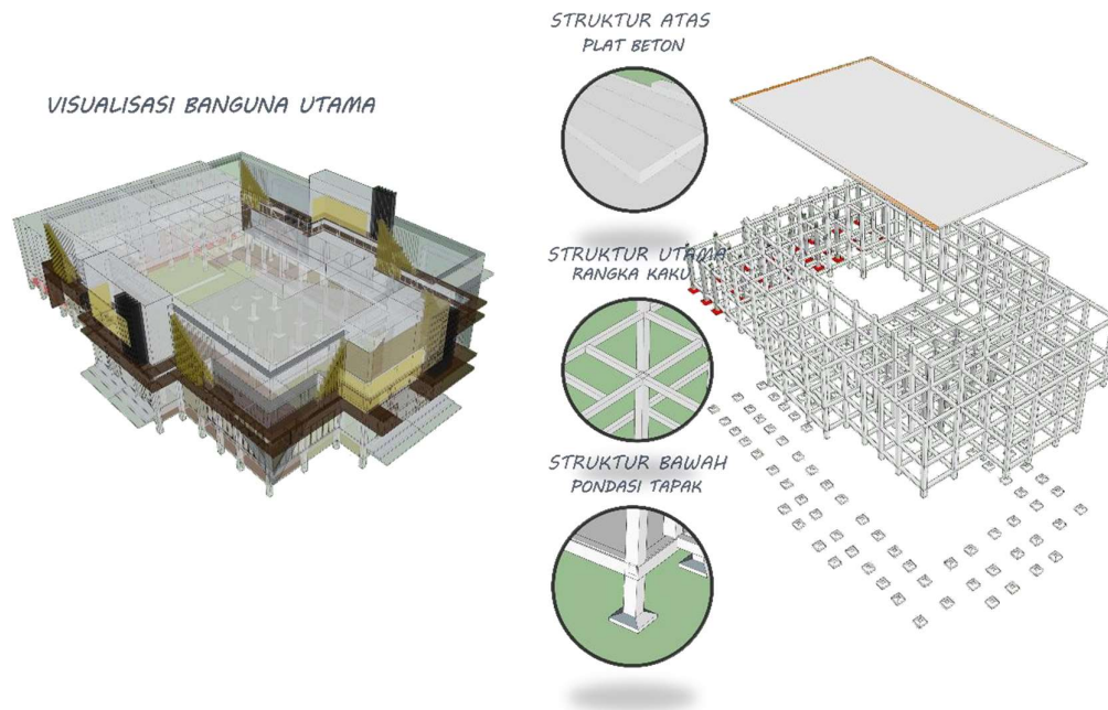
Gambar 5.4. Konsep Struktur Gedung Pertunjukan Seni
