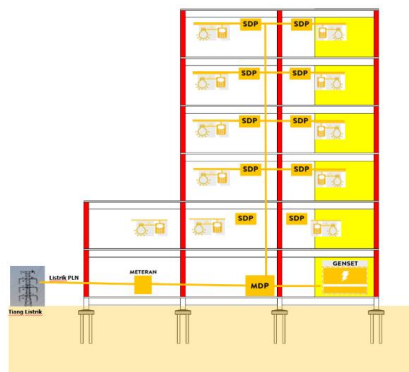
Gambar 13 sistem elektrikal
