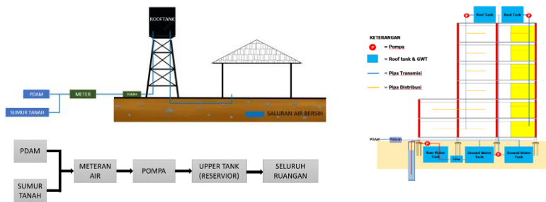
Gambar 9 sistem air bersih Sumber: Analisis peribadi, 2023
