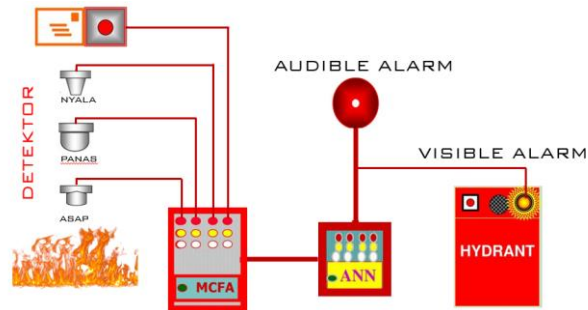
Gambar 14 sistem kebakaran Sumber: Analisis pribadi, 2023
