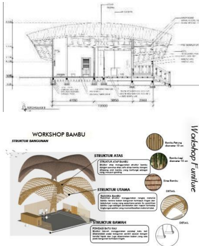
Gambar 7. Struktur Utama & Atas Sumber: Dokumen Pribadi, 2023
