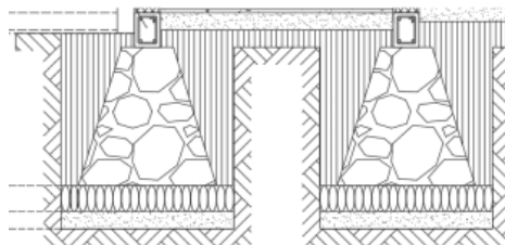
Gambar 6. Struktur Bawah Sumber: Dokumen Pribadi, 2023
