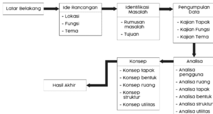
Gambar 1. Metode Perancangan
