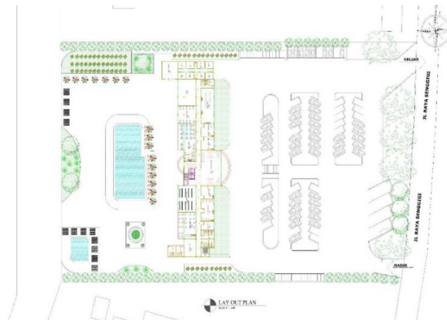
Gambar 17 Layout plan Sumber: Analisa Pribadi, 2023
