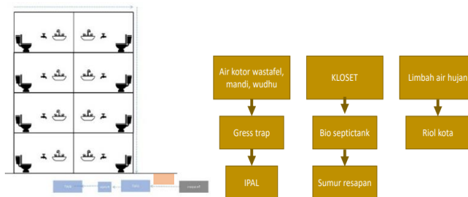
Gambar 11. Sistem air kotor Sumber: Analisa Pribadi, 2023
