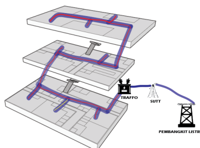
Gambar 7. Jaringan Listrik
