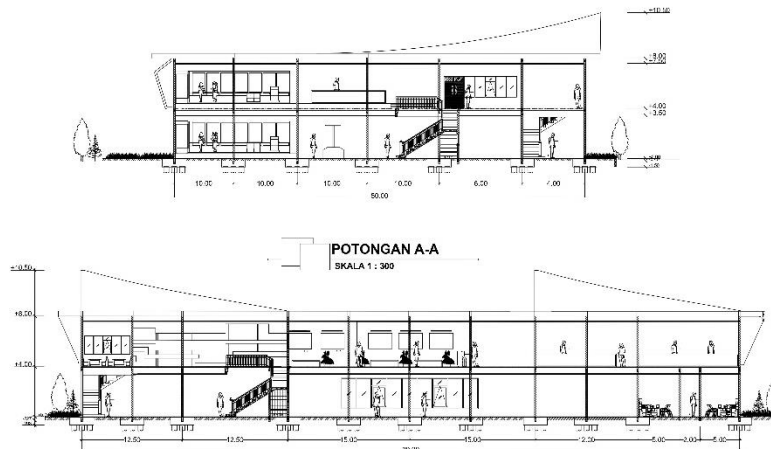
Gambar 14. Sumber: Data Pribadi Potongan
