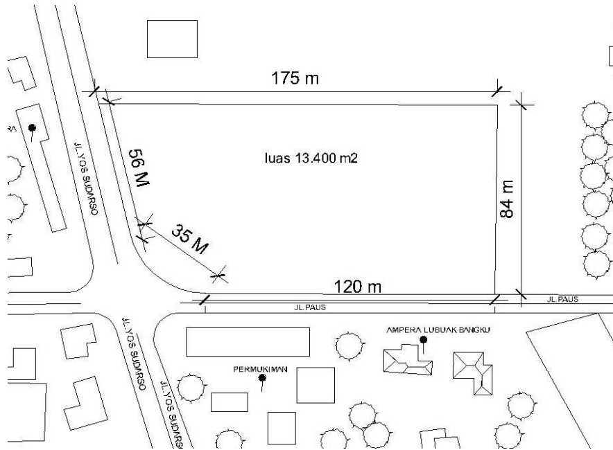
Gambar 2. Sumber: Dokumen Pribadi Dimensi Tapak
