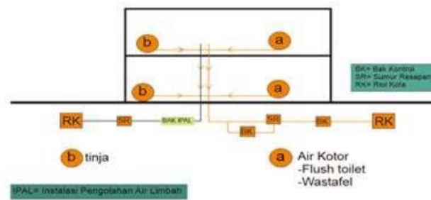
Gambar 17 Skema air kotor
