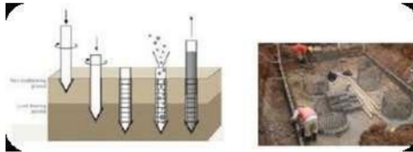
Gambar 13 Pondasi borepile
