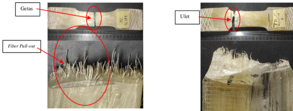
Gambar 5. (a) Foto makro serat 10 % sebelum alkalisasi NaOH (b) Foto makro serat 10 % setelah alkalisasi NaOH 5%
