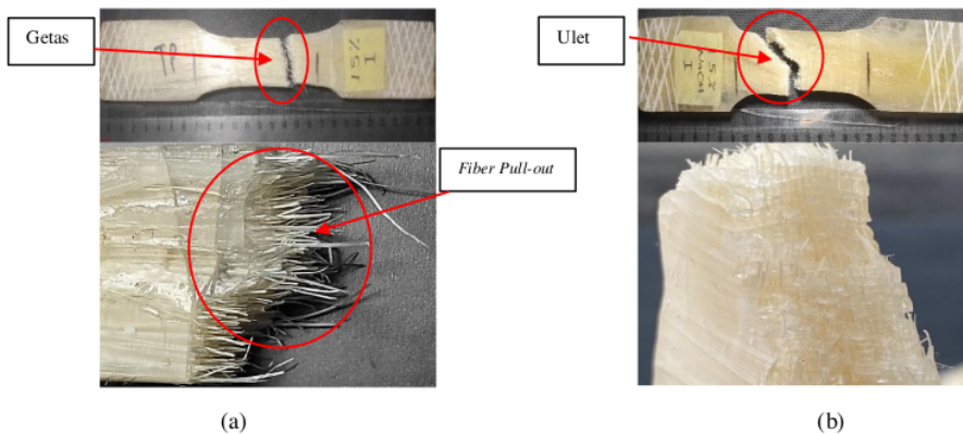
Gambar 6. (a) Foto makro serat 15 % sebelum alkalisasi NaOH (b) Foto makro serat 15 % setelah alkalisasi NaOH 5%
