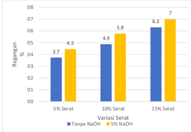
Gambar 3. Perbandingan fraksi volume serat dan regangan tanpa NaOH dan 5% NaOH
