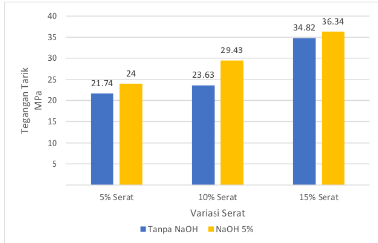
Gambar 2. Perbandingan fraksi volume serat dan tegangan tanpa NaOH dan 5% NaOH
