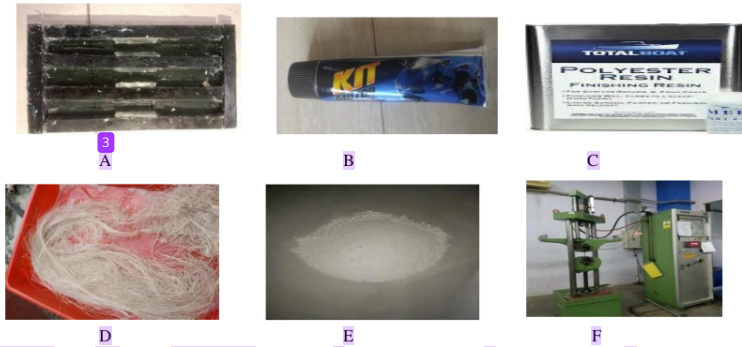
Gambar 1. Alat dan Bahan Penelitian A). Cetakan, B). Pelumas Cetakan, C). Resin Polyester, D). Serat Eceng Gondok, E). Zinc Oxide, F). Alat Uji Tarik
