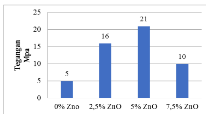
Gambar 3. Grafik Tegangan Maksimal
