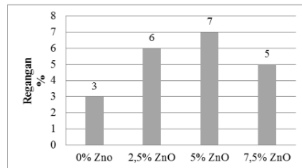
Gambar 4. Grafik Regangan
