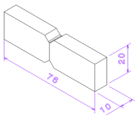
Gambar 12. Ukuran spesimen uji standar ASTM D5379-98
