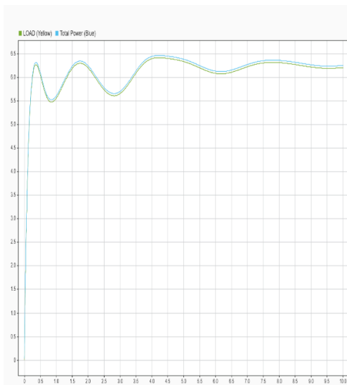
Gambar. 15 Grafik beban dan daya PLTS
