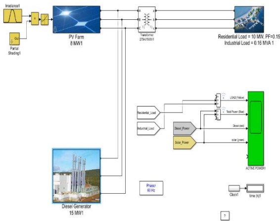
Gambar. 10 PV Array PLTS dan generator diesel
