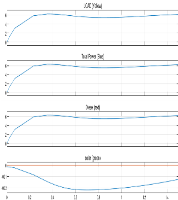
Gambar. 12 Grafik simulasi MATLAB
