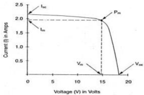
Gambar. 3 Grafik I-V curve
