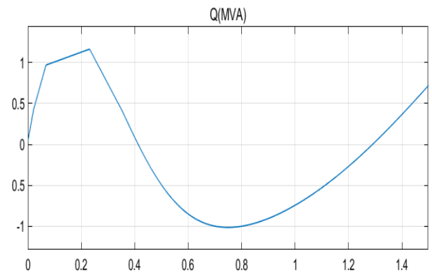
Gambar. 13 Grafik daya aktif dan daya reaktif generator diesel
