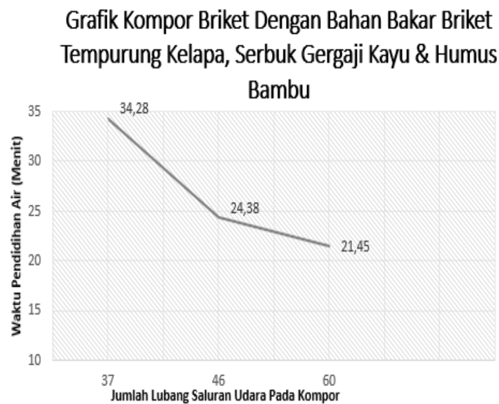
Grafik 3 Hasil Pengujian Kompor Briket Dengan Briket Tempurung Kelapa, Serbuk Gergaji Kayu Dengan Campuran Humus Bambu
