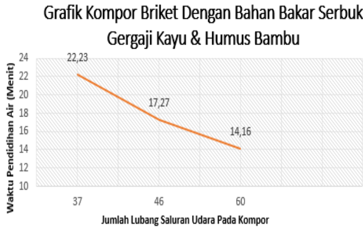
Grafik 2 Hasil Pengujian Kompor Briket Dengan Briket Serbuk Gergaji Kayu Dengan Campuran Humus Bambu
