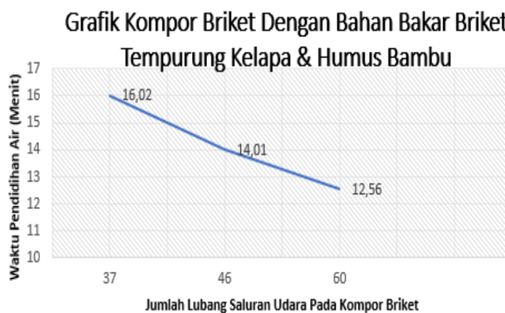
Grafik 1 Hasil Pengujian Kompor Briket Dengan Briket Tempurung Kelapa Dengan Campuran Humus Bambu
