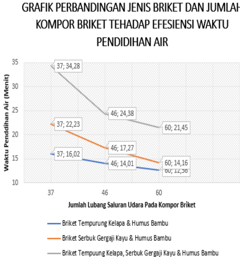
Grafik 4 Perbandingan Jenis Briket Dan Jumlah Lubang Udara Pada Kompor Briket Terhadap Efisiensi Waktu Pendidihan Air
