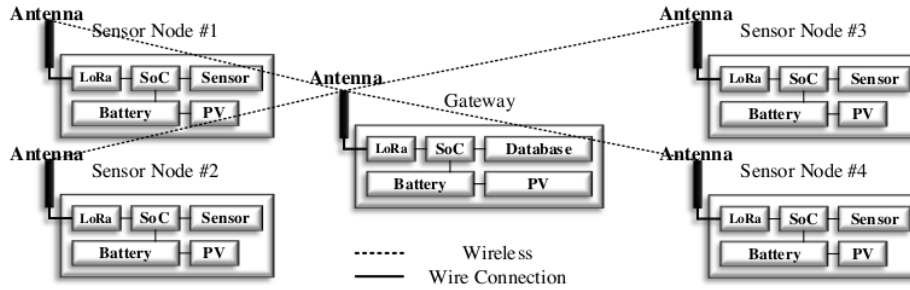
Gambar 1 Topologi Jaringan Star
