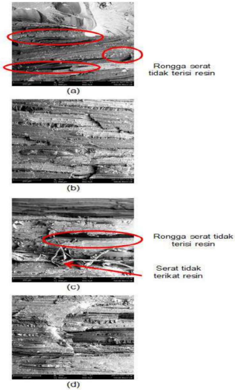
Gambar 5.9 Hasil foto SEM pembesaran 300x pada ikatan komposit antara serat kulit pohon waru dan jenis resin sintetis, (a) Resin poliester BTQN 157, (b) Resin bisphenol LP-1Q-EX (c) Resin epoksi R-802, (d) Resin Epoksi
