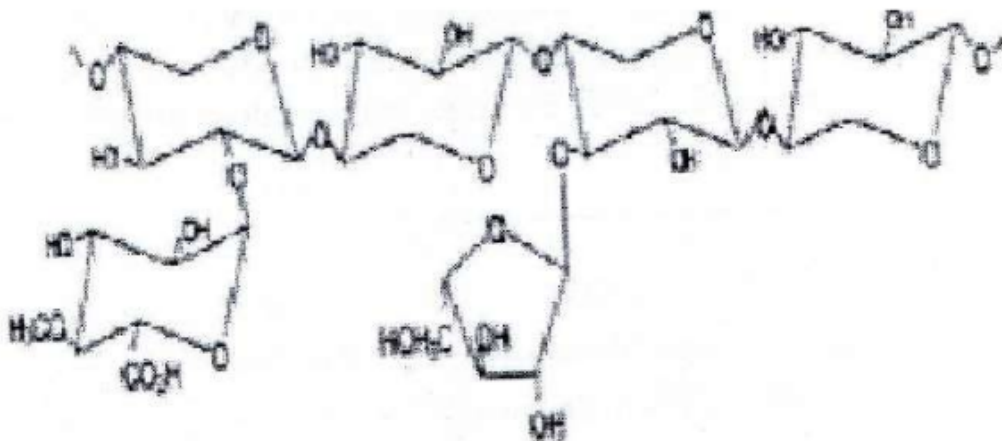
Gambar 2.4 Struktur dasar lignoselulosa hemiselulosa
