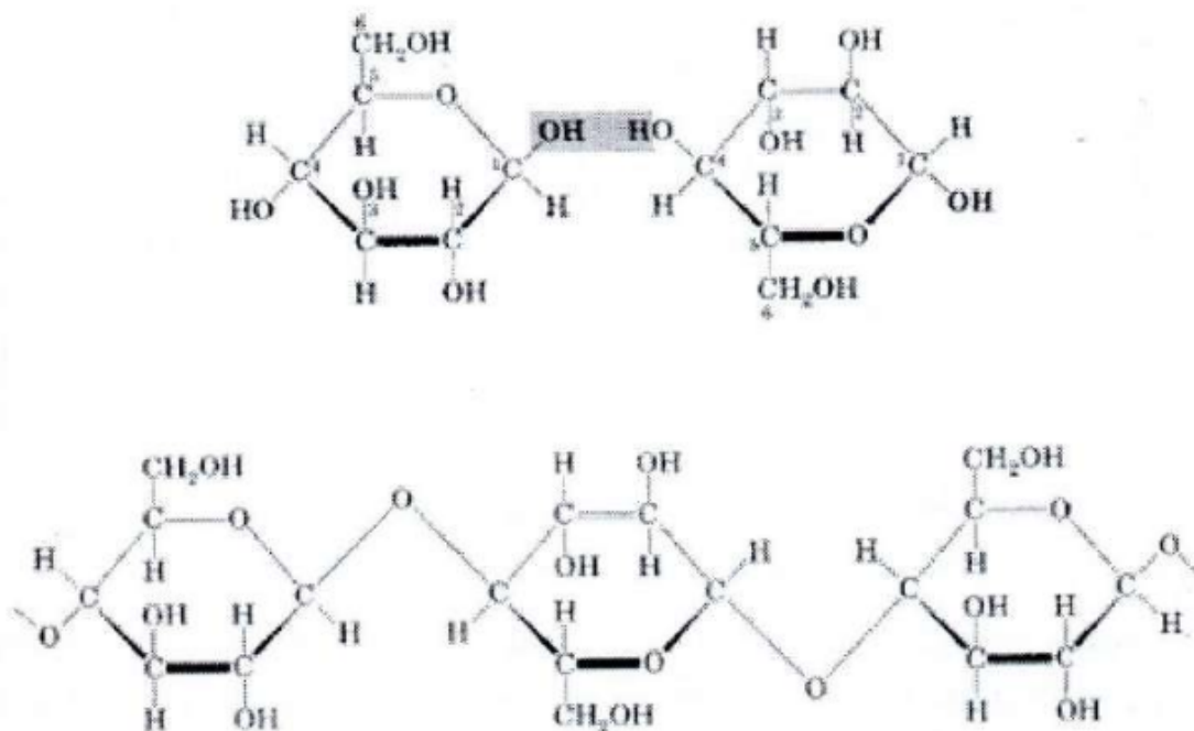
Gambar 2.1 Struktur selulosa
