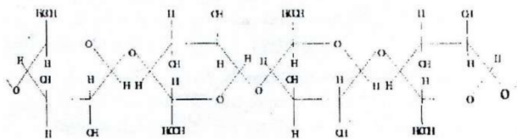
Gambar 2.2 Stuktur molekul selulosa
