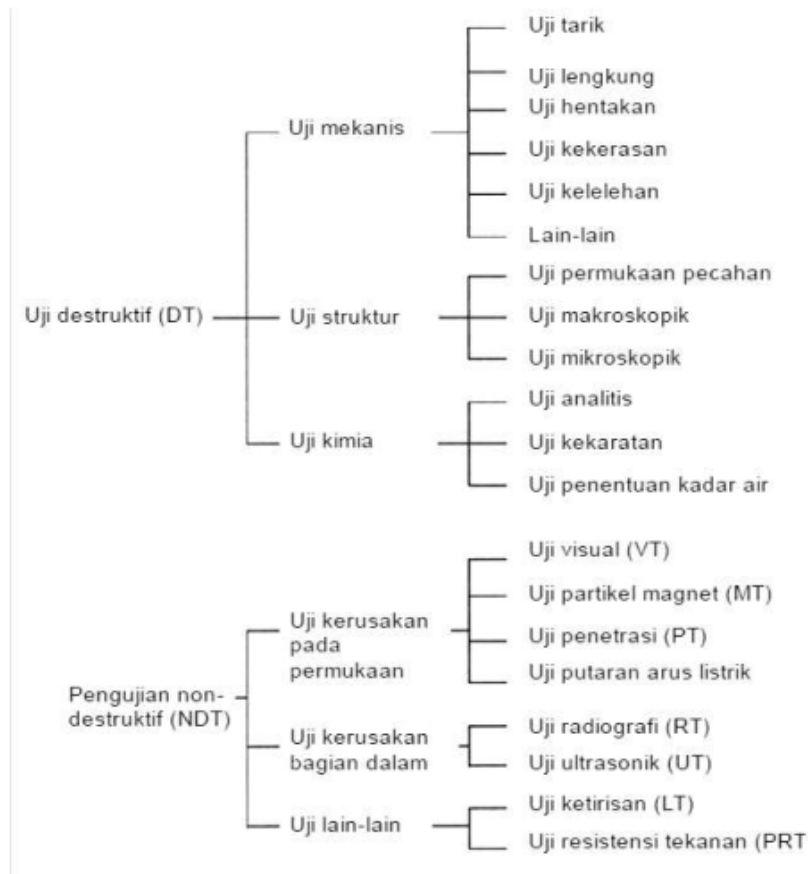
Gambar 4.1 Klasifikasi metode pengujian komposit (Sumber: Sunaryo, 2008; 442)
