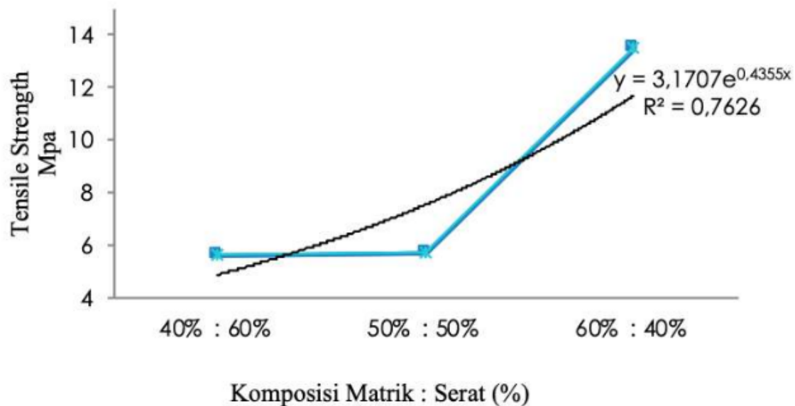
Gambar 5.2 Grafik Uji Tarik Komposit
