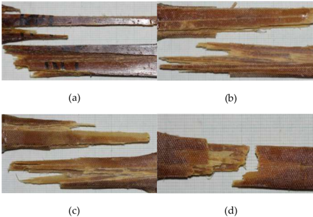
Gambar 5.10 Patahan uji tarik komposit serat kulit pohon waru variasi jenis resin, (a) resin poliester BTQN 157, (b) resin bisphenol LP-1Q-EX, (c) resin epoksi R-802, (d) resin epoksi A dan B
