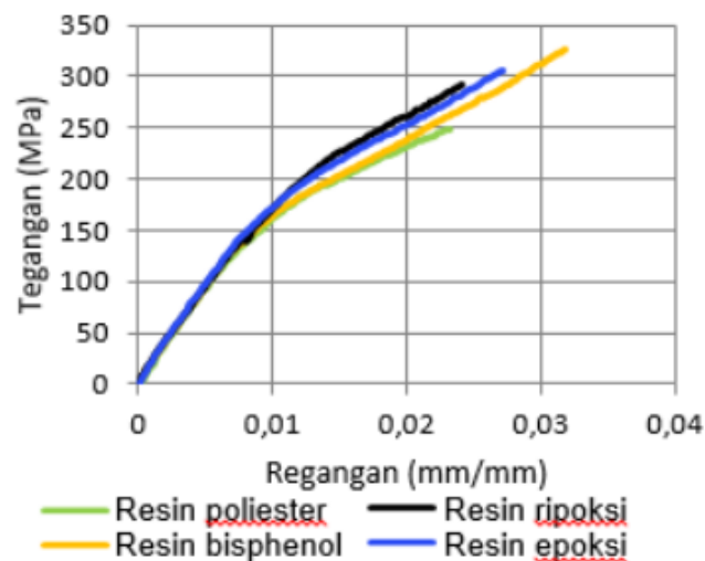
Gambar 5.6 Tegangan-regangan komposit serat waru variasi jenis resin
