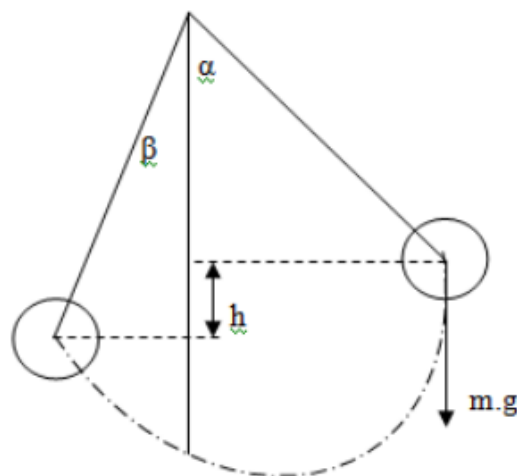
Gambar 4.8 Mekanisme pengujian impak (Sumber: modul praktikum material teknik 2 ITN Malang)
