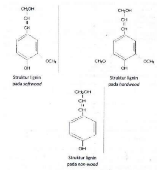
Gambar 2.5 Struktur lignin
