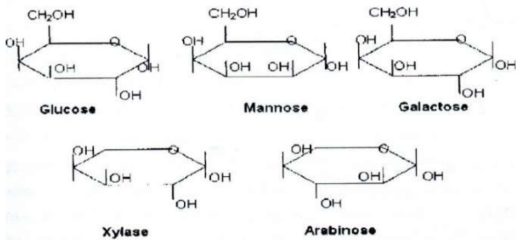
Gambar 2.3 Struktur hemiselulosa
