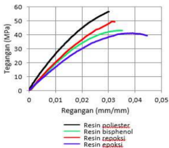
Gambar 5.8 Tegangan-regangan jenis resin tanpa serat
