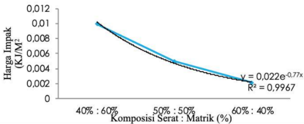
Gambar 5.4 Grafik Harga Impak Komposit
