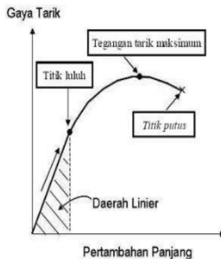
Gambar 4.3 Gambaran singkat uji tarik
