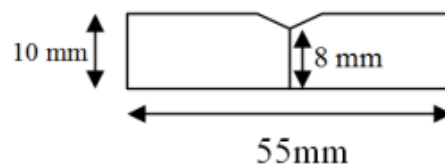
Gambar 4.9 Spesimen uji impact sesuai standar ASTM 5942-96
