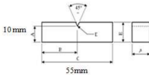
Gambar 6.1 Desain spesimen uji
