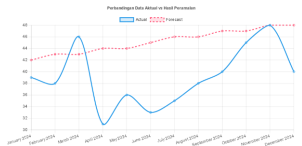
Gambar 2. Tampilan grafik peramalan
