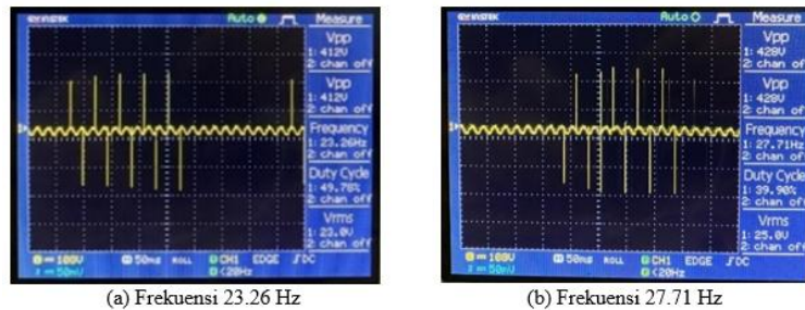
Gambar 5. Tampilan Gelombang Frekuensi 23 Hz dan 27 Hz Pada Osiloscope
