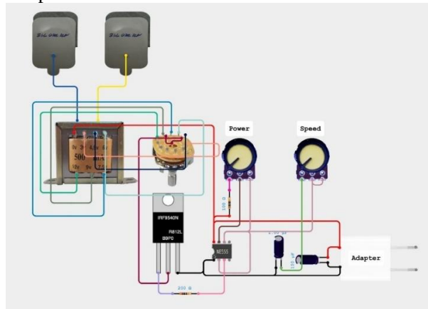
Gambar 2. Skematik Sistem Stimulator
