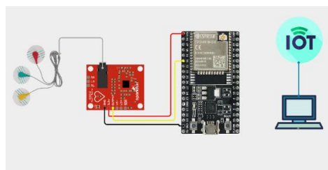
Gambar 3. Skematik Sistem EMG
