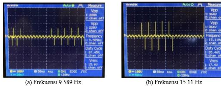
Gambar 4. Tampilan Gelombang Frekuensi 9 Hz dan 15 Hz Pada Osiloscope
