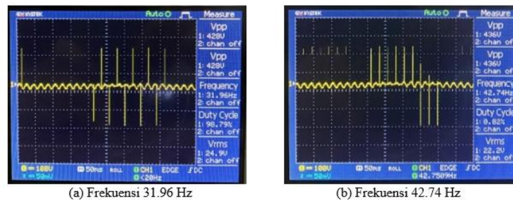
Gambar 6. Tampilan Gelombang Frekuensi 231 Hz dan 42 Hz Pada Osiloscope
