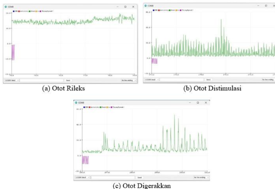
Gambar 7. Hasil Serial Ploter Arduino IDE Monitoring Otot Ketika Rileks (a), Distimulasi Listrik (b), dan Digerakkan (c)
