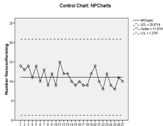
Gambar 1. Grafik Peta Kendali NP ( Sumber : Pengolahan Data )
