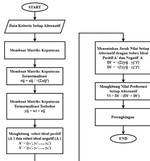
Gambar 1. Metode TOPSIS
