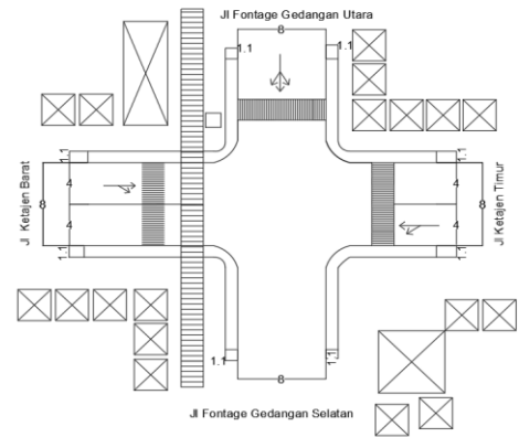
Gambar 3. Geometrik Simpang
