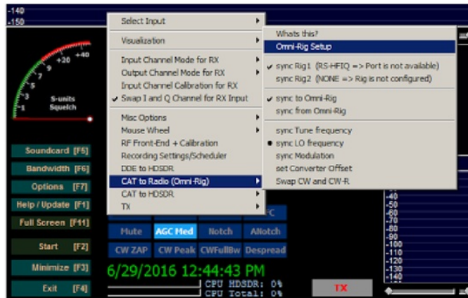
Gambar 4.7 Konfigurasi Omni-Rig
