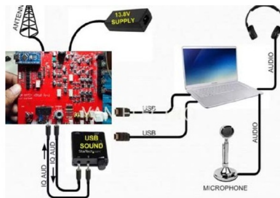
Gambar 4.1 Diagram rangkaian uji
