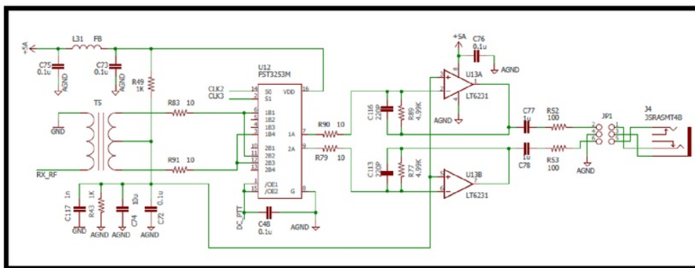
Gambar 3.3 Rangkaian Multiplexer
