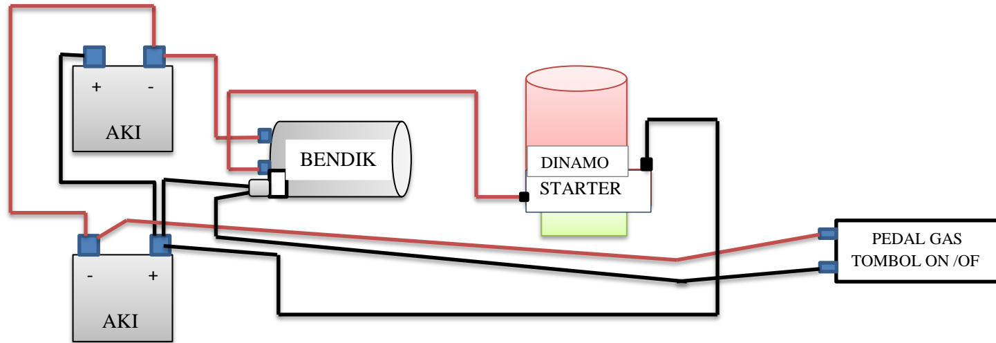
Gambar rangkaian kelistrikan electric longboard
