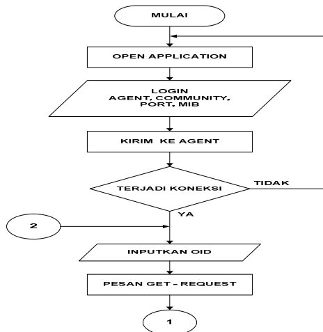
Gambar 6. Manajer SNMP.
