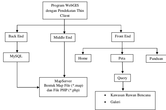
Gambar 3. Alir Program SIG WEB
