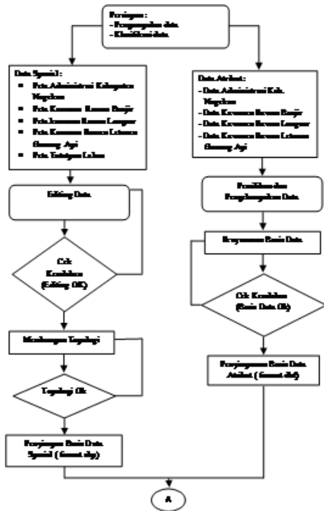
Gambar 1. Alir Pekerjaan Penelitian
