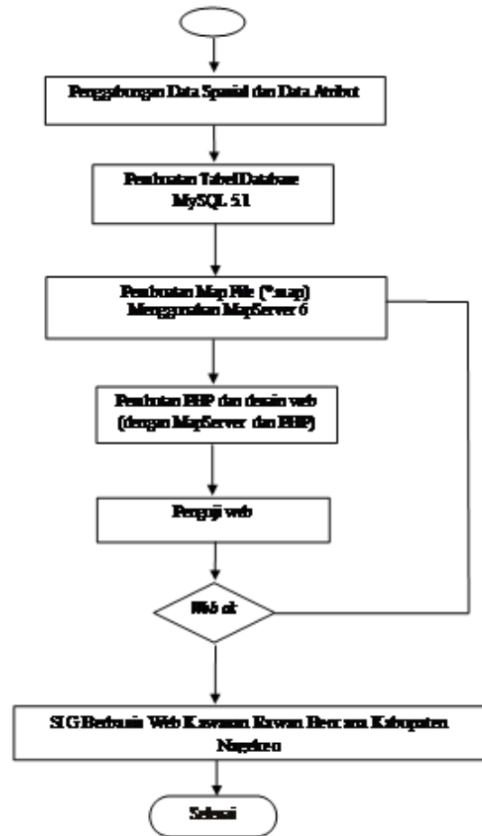
Gambar 2. Alir Pekerjaan Lanjutan
